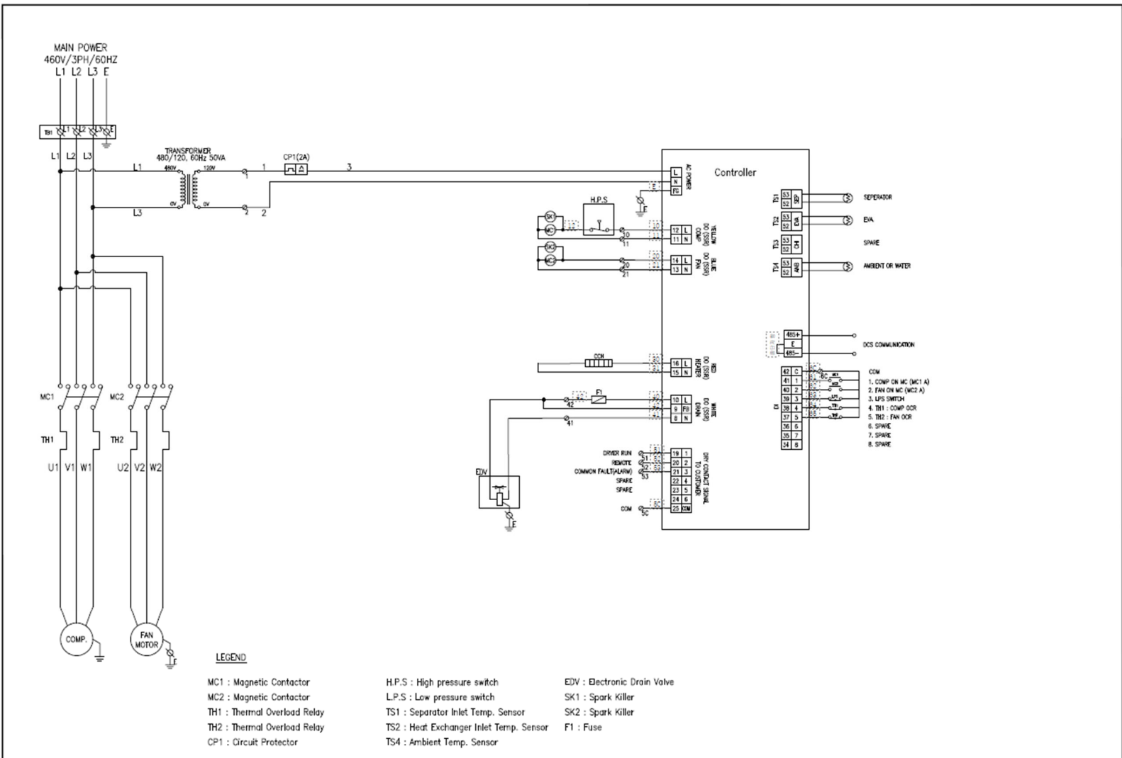
Figure 9C Models: DFXA 3.1-A, DFXA 4.5-A, DFXA 5.5-A
